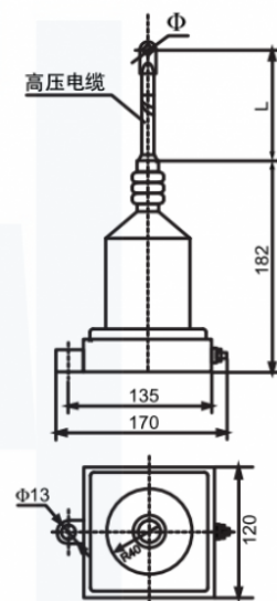
35kV系统户内型TBP安装尺寸
