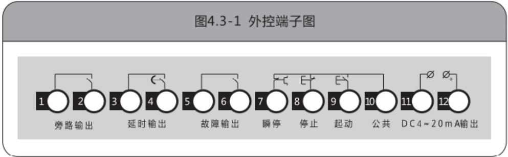
4.5软起动器的外控端子说明: 图4.3-1外控端子图
