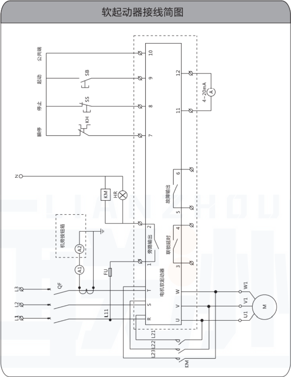
4.5软起动器的外控端子说明: 图4.3-1外控端子图
