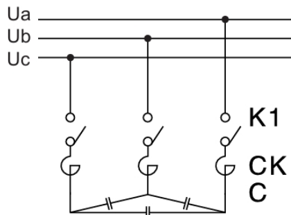
与三相共补偿电容器连接
