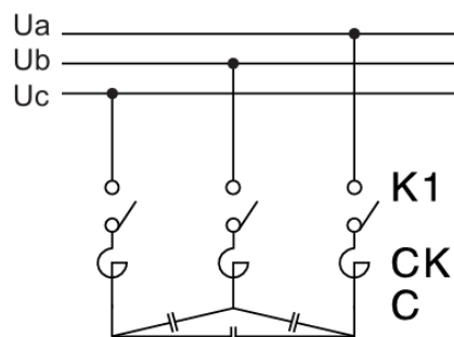
与三相共补偿电容器连接
