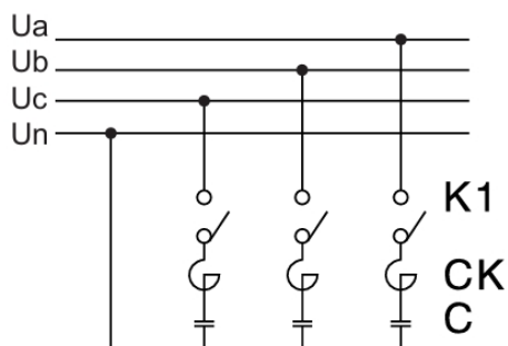
与分相补偿电容器连接
